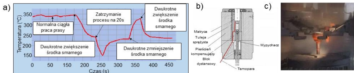
Rys. 5a) Zmian temperatury w matrycy podczas kucia z zaznaczonymi najczęściej występującymi zakłóceniami w procesie, b) schemat zamontowania termopary w narzędziu, c) widok przenoszonych odkuwek na prasie transferowej
